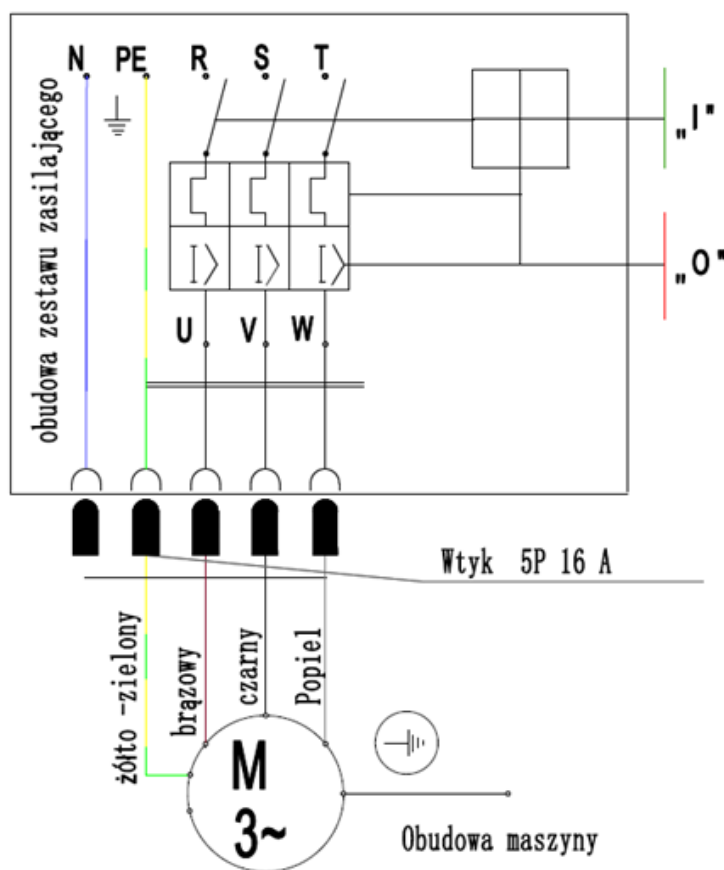
Rysunek 5 Schemat elektryczny
